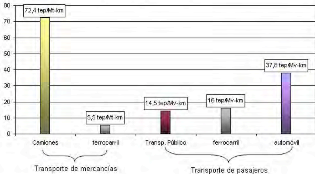
Figura 26. Consumo energético específico tep/Mt-km y tep/Mv-km. Unión Europea.
