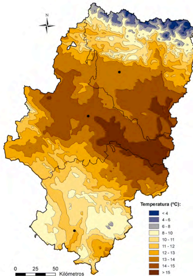
Figura 9. Temperatura media anual del periodo 1971-2000. Atlas Climático de Aragón.
