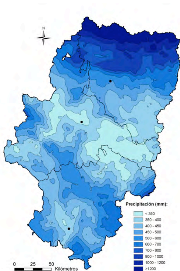
Figura 7. Precipitación media anual del periodo 1971-2000. Atlas Climático de Aragón.
